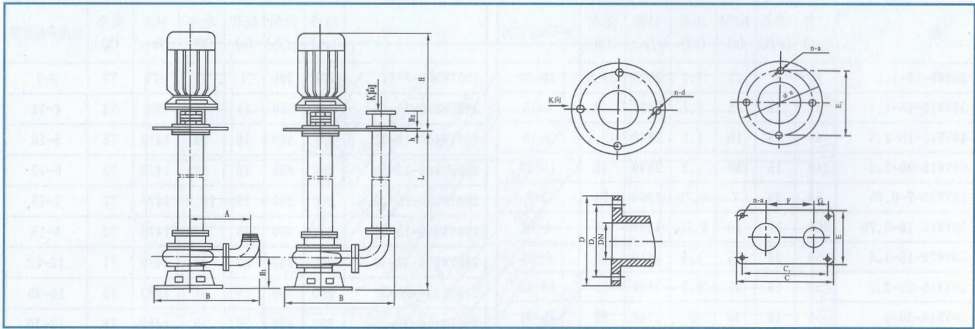
安装尺寸表
