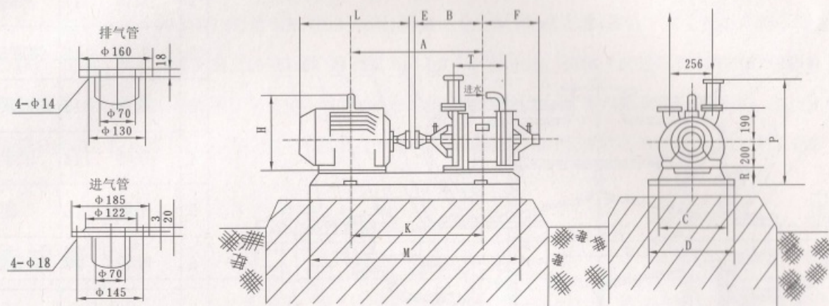
图7 SZ-1、SZ-2水环式真空泵外形及安装图
