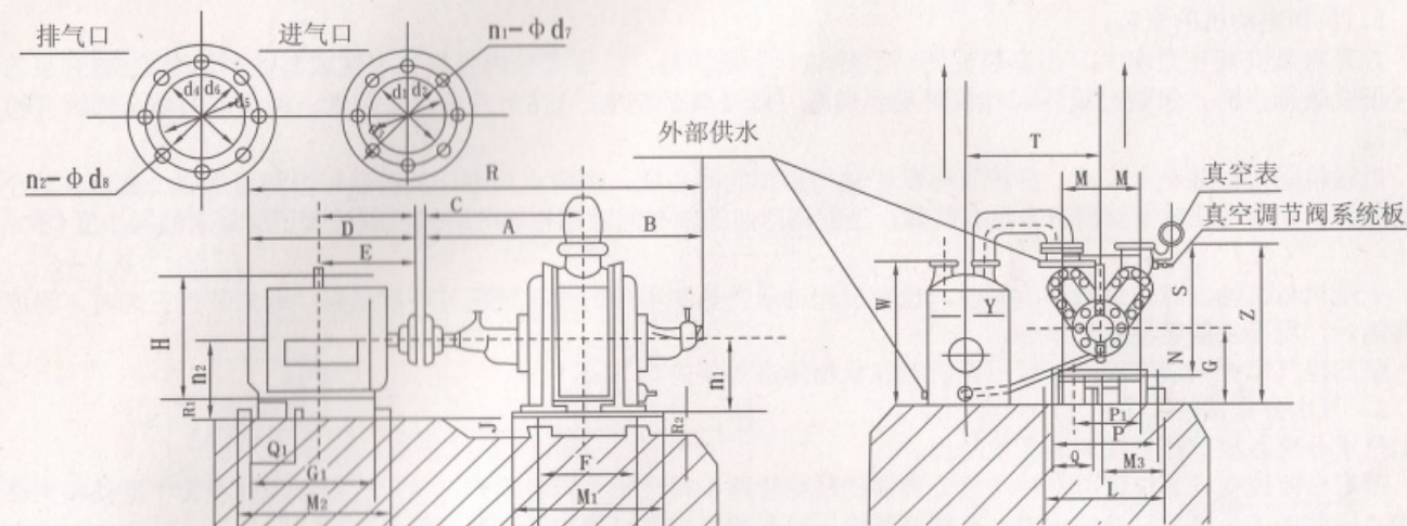
图10 SZ-4水环式真空泵外形安装图
