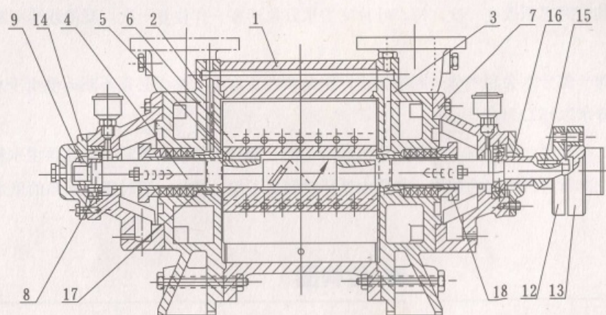
图3 SZ-1、SZ-2型水环式真空泵及压缩机结构图
