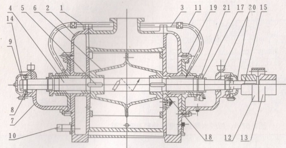
图4 SZ-3、SZ-4型水环式真空泵及压缩机结构图
