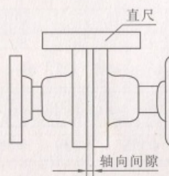
图12 校正同心度的方法
