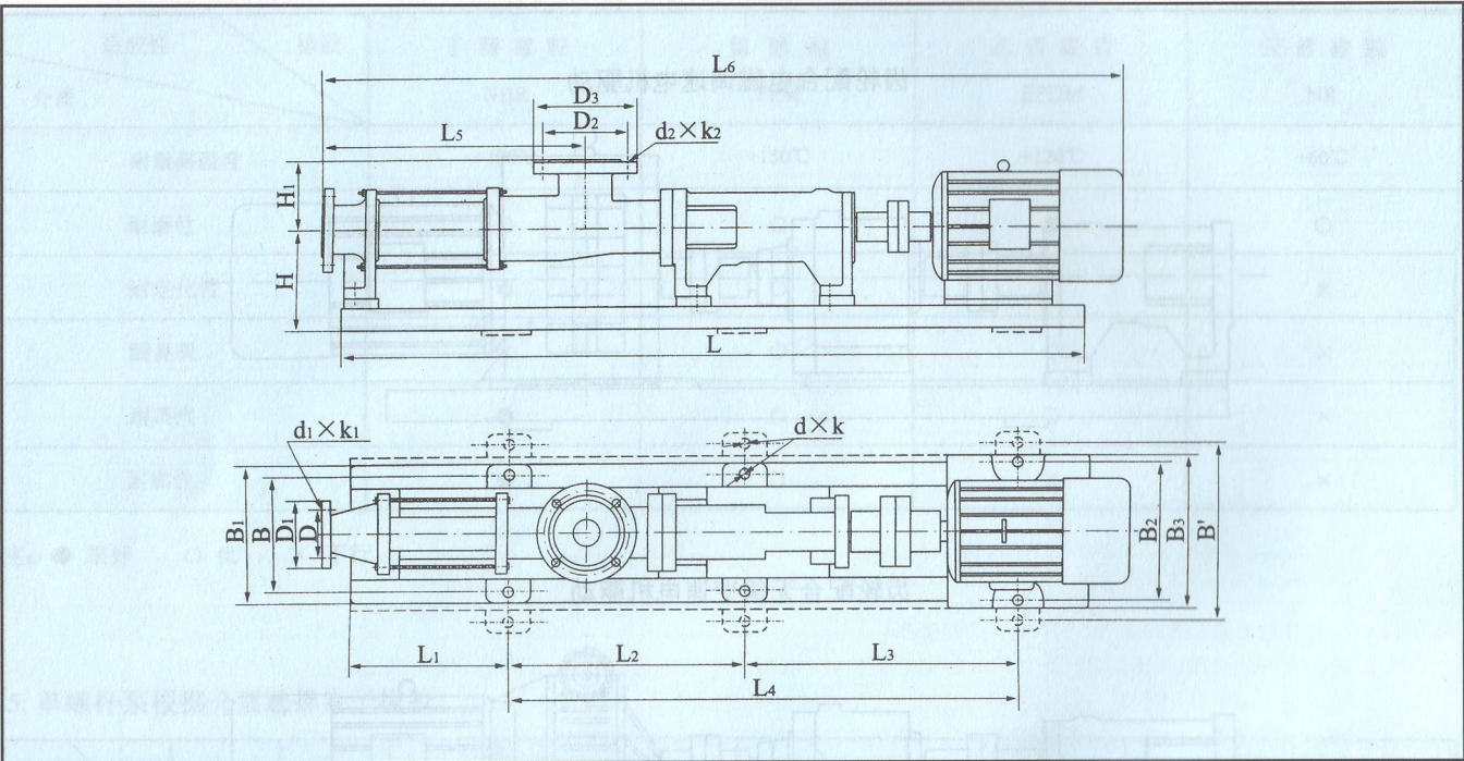
泵的安裝尺寸(固定轉速時的尺寸, 特定轉速的安裝尺寸在訂貨時附給)
