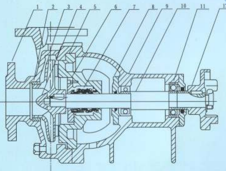
FB、AFB型结构图
